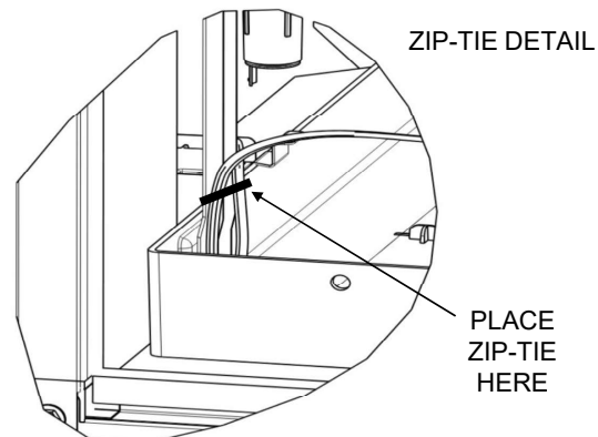
ZIP-TIE DETAIL
