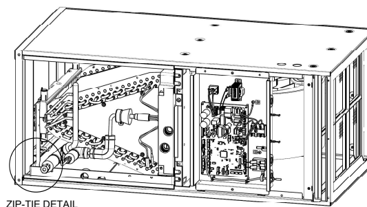
ZIP-TIE DETAIL
